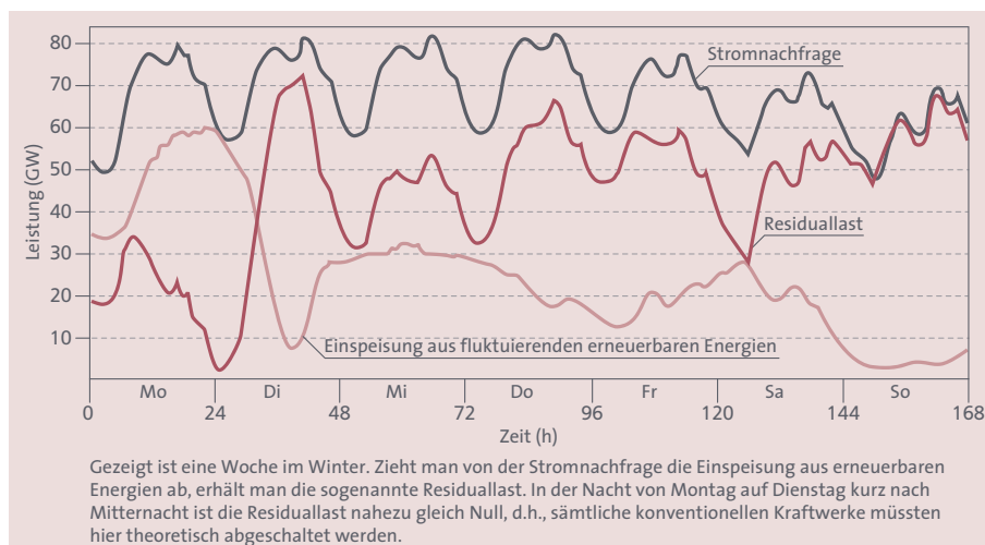
ABB. 1 ZUSAMMENHANG ZWISCHEN STROMNACHFRAGE UND RESIDUALLAST
